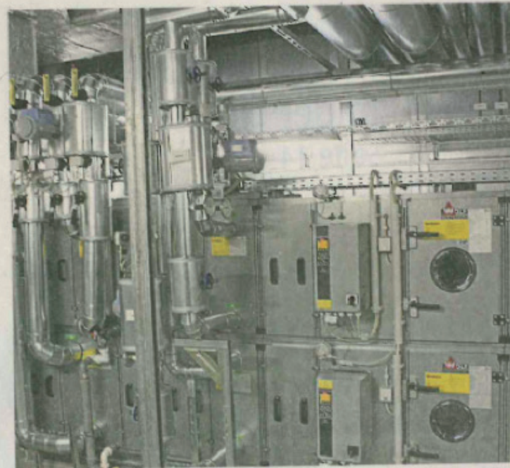
Die Anlage mit integriertem Gegenstrom-Schicht-Wärmetauschersystem sorgt für hohe Energieeffizienz. Foto: Kliniken Maria Hilf
